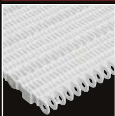
50-401 Лента с открытой поверхностью (61 %). Для охлаждения и заморозки продукции
