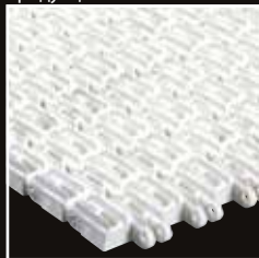
25-402 Лента с ребристой поверхностью (29%) Для транспортировки продукции, требующей небольшой площади контакта с поверхностью ленты
