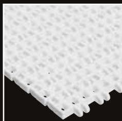
25-400 Лента с открытой поверхностью (29%). Для процессов охлаждения/заморозки и мойки продукции
