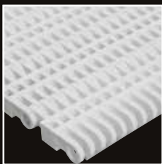
50-100 Лента с открытой поверхностью (27 %). Для транспортировки продукции большого веса
