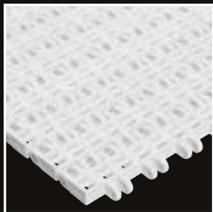
25-411 Лента с открытой поверхностью (26 %). Для процесса бланширования и изготовления лапши
