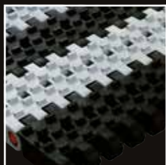
50-930 Ленты с перфорированной поверхностью (13%) и с выступающими ребрами H=3мм. Для автомобильной промышленности
